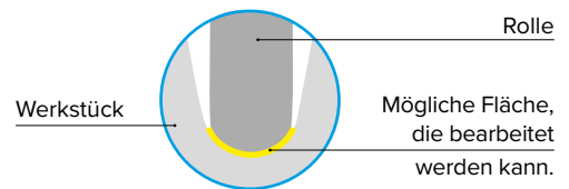
Detaildarstellung Kernradius
